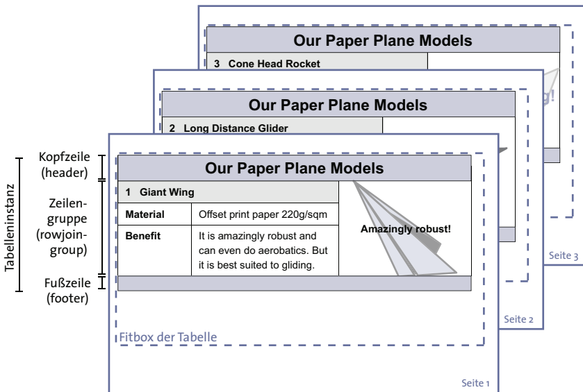
Abb. 8.37 Tabelle besteht aus Tabelleninstanzen, die in jeweils einer Fitbox platziert werden.
